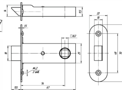
ЗАЩЕЛКА МЕЖКОМНАТНАЯ ЗЩ2.03
