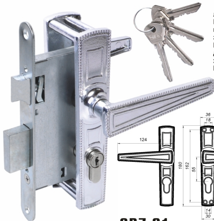
ЗАМОК ВРЕЗНОЙ ЦИЛИНДРОВЫЙ ТИП ЗВ7.01
