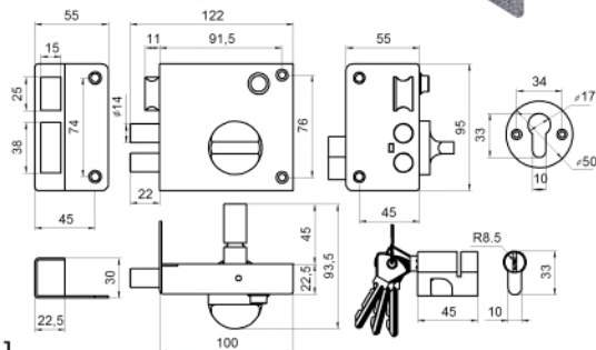
ЗАМОК НАКЛАДНОЙ ТИП ЗН-3
