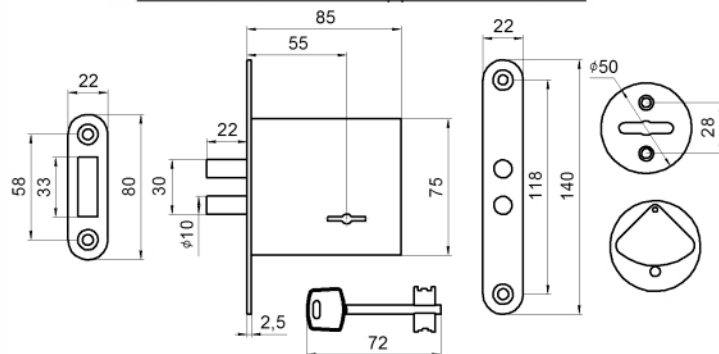
ЗАМОК ВРЕЗНОЙ СУВАЛЬДНЫЙ ТИП ЗВ8-4 2Р
