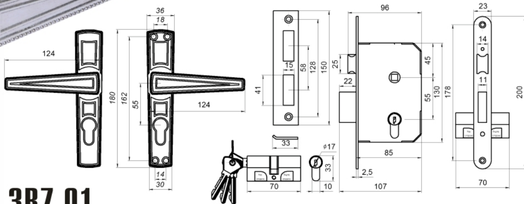
ЗАМОК ВРЕЗНОЙ ЦИЛИНДРОВЫЙ ТИП ЗВ7.01
