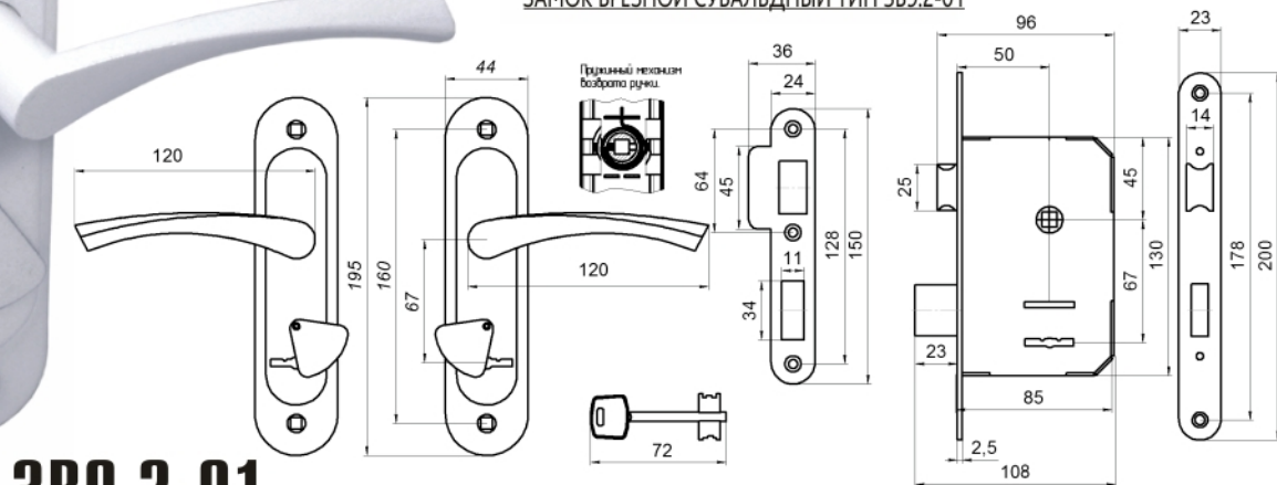
ЗАМОК ВРЕЗНОЙ СУВАЛЬДНЫЙ ТИП ЗВ9.2-01
