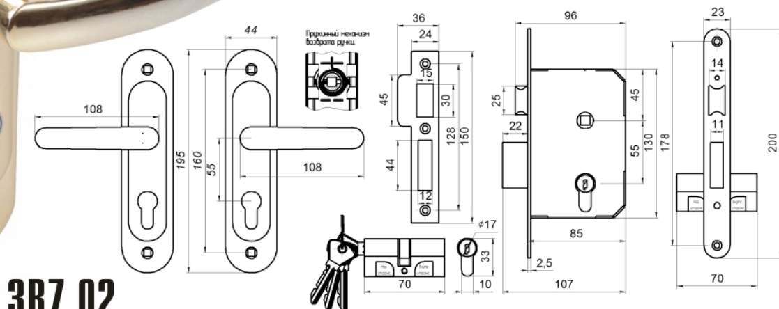
ЗАМОК ВРЕЗНОЙ ЦИЛИНДРИЧЕСКИЙ ТИП 3В7.02
