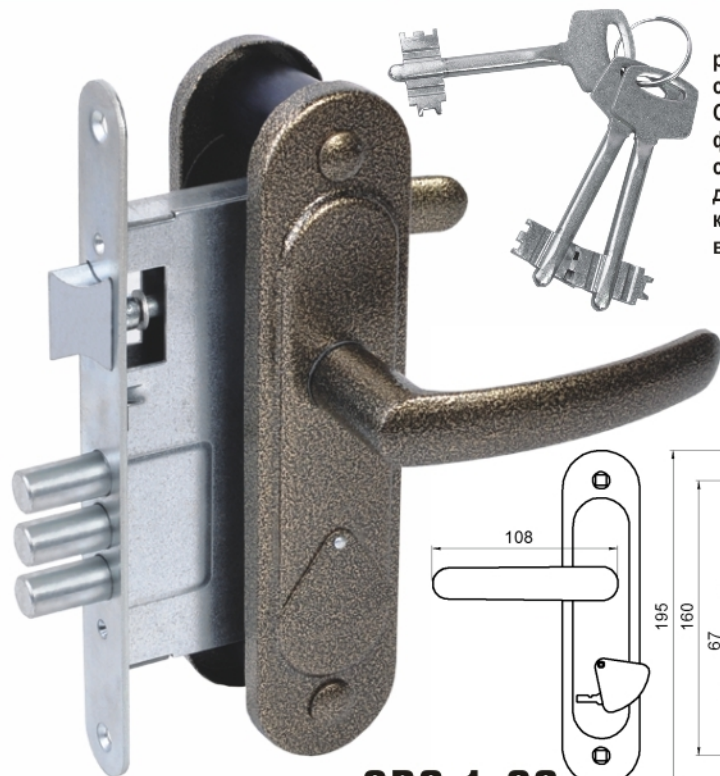
ЗАМОК ВРЕЗНОЙ СУВАЛЬДНЫЙ ТИП ЗВ9.1-02
