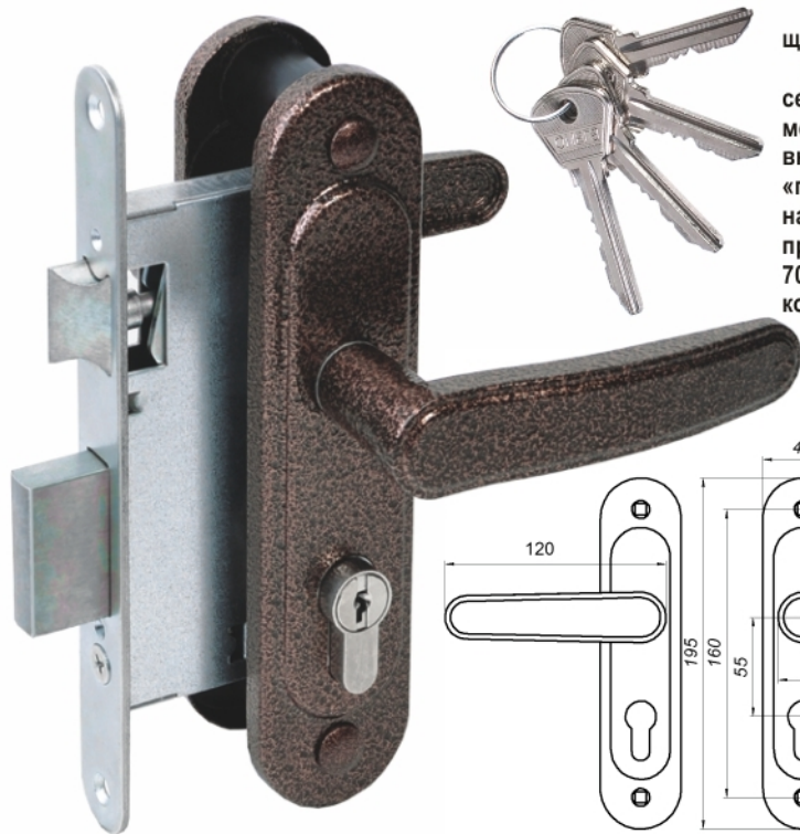
ЗАМОК ВРЕЗНОЙ ЦИЛИНДРИЧЕСКИЙ ТИП ЗВ7.03
