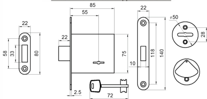
ЗАМОК ВРЕЗНОЙ СУВАЛЬДНЫЙ ТИП 3В8-4
