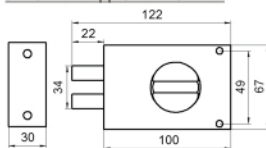
ЗАМОК НАКЛАДНОЙ ТИП ЗН-1 2Р
