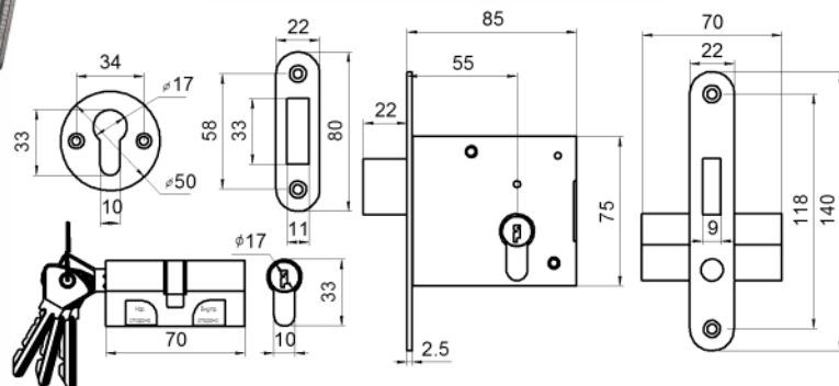
ЗАМОК ВРЕЗНОЙ ЦИЛИНДРИЧЕСКИЙ ТИП ЗВ1
