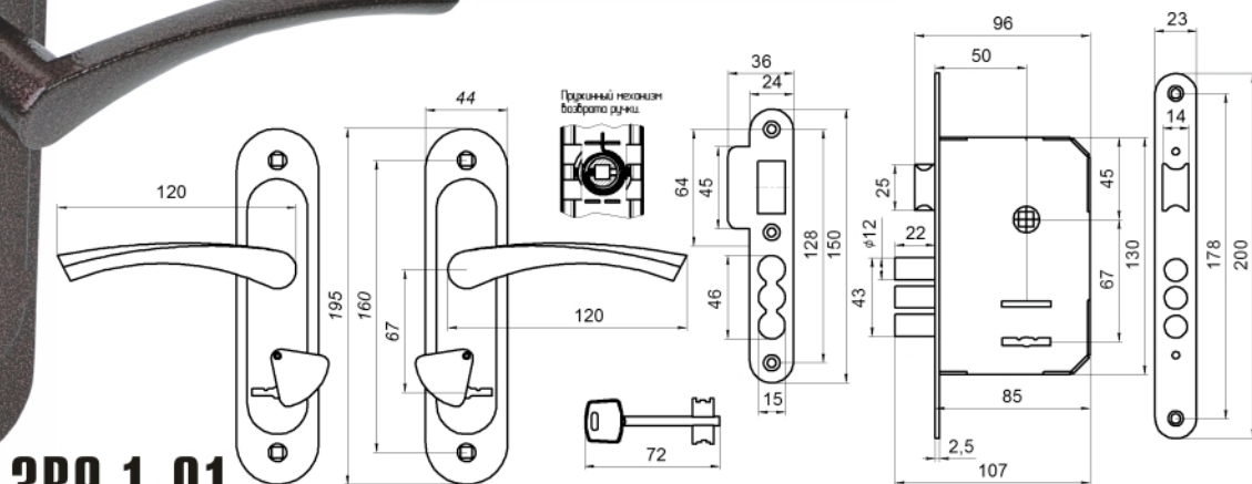
ЗАМОК ВРЕЗНОЙ СУВАЛЬДНЫЙ ТИП 3В9.1-01
