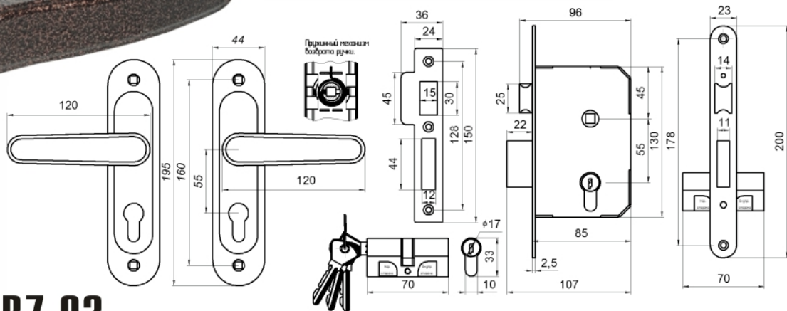
ЗАМОК ВРЕЗНОЙ ЦИЛИНДРИЧЕСКИЙ ТИП ЗВ7.03
