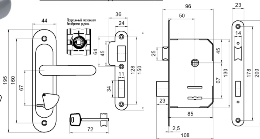
ЗАМОК ВРЕЗНОЙ СУВАЛЬДНЫЙ ТИП ЗВ9.2-02
