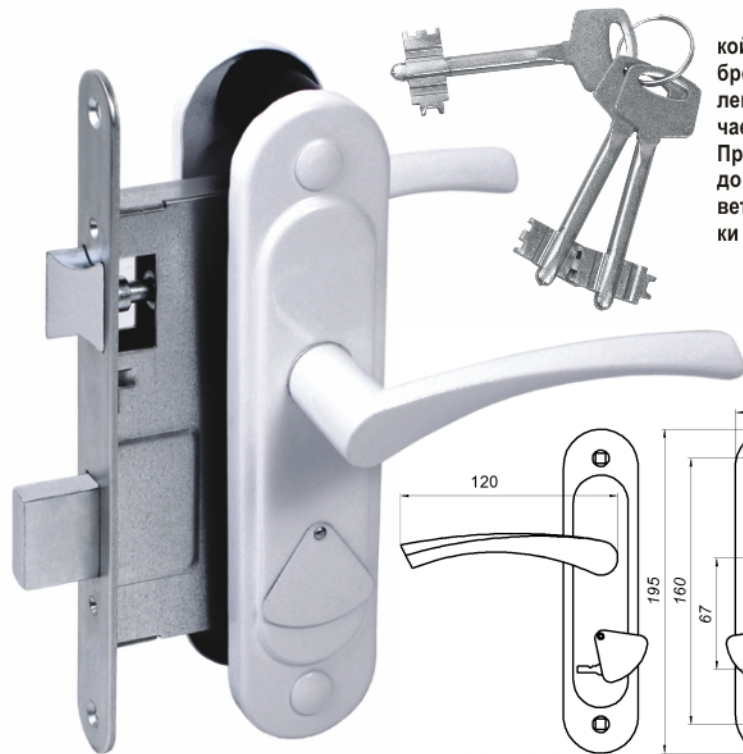
ЗАМОК ВРЕЗНОЙ СУВАЛЬДНЫЙ ТИП ЗВ9.2-01
