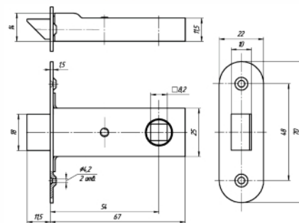
ЗАЩЕЛКА МЕЖКОМНАТНАЯ ЗЩ2.05
