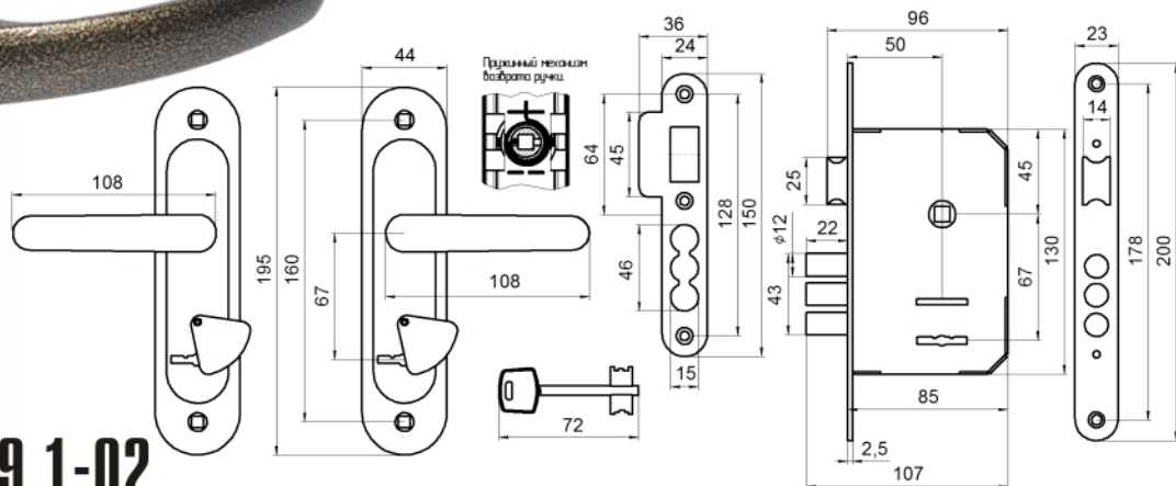
ЗАМОК ВРЕЗНОЙ СУВАЛЬДНЫЙ ТИП ЗВ9.1-02
