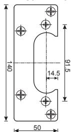
Крепежная пластина DH-1130-111*29*6
