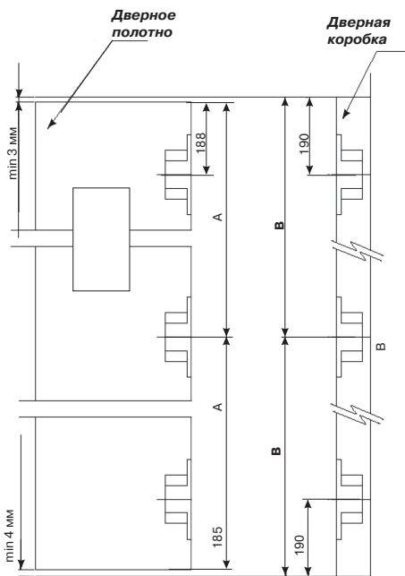
Рис. 4 Схема разметки дверного полотна и дверной коробки для установки петли.
